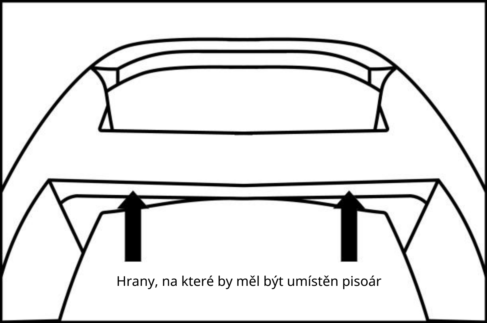
Nainstalujte držáky pro upevnění pisoáru na stěnu
