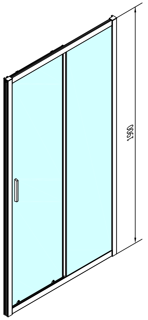
EL1815R
