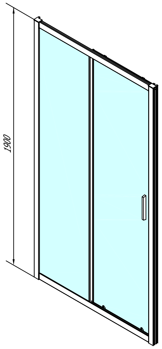
EL1815L
