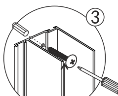
Šroub M4x35
