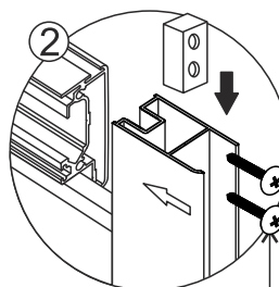
Šroub M4x35
