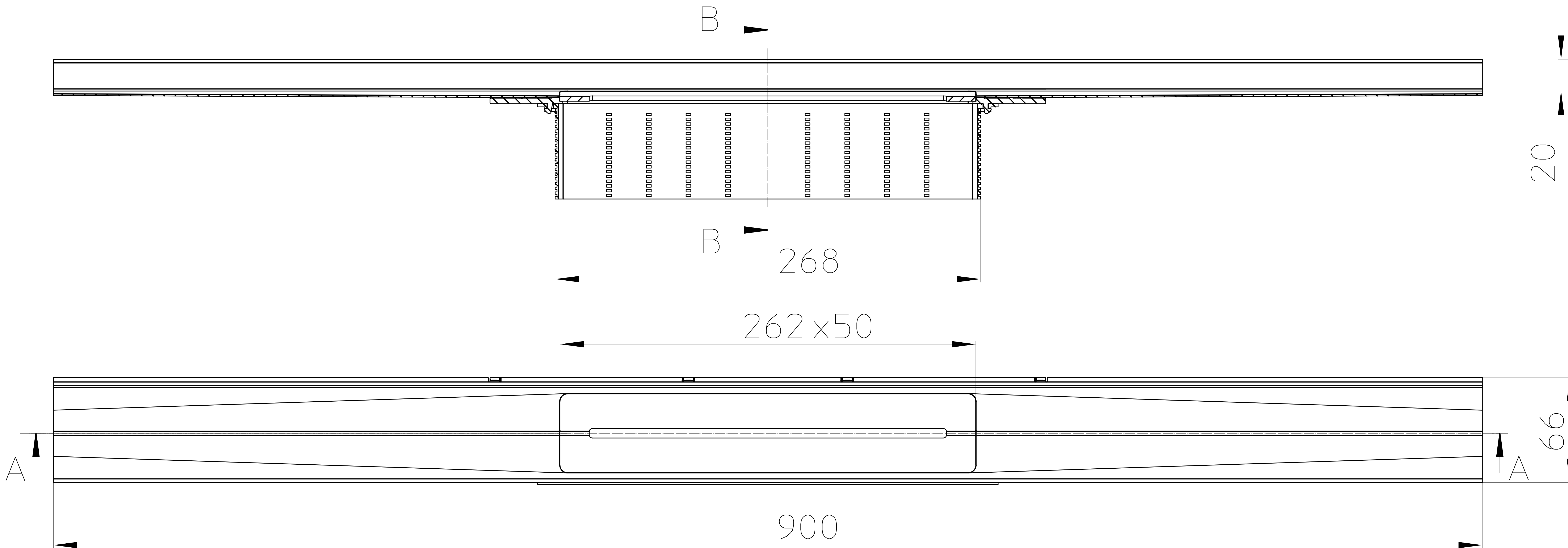
Schnitt A-A
