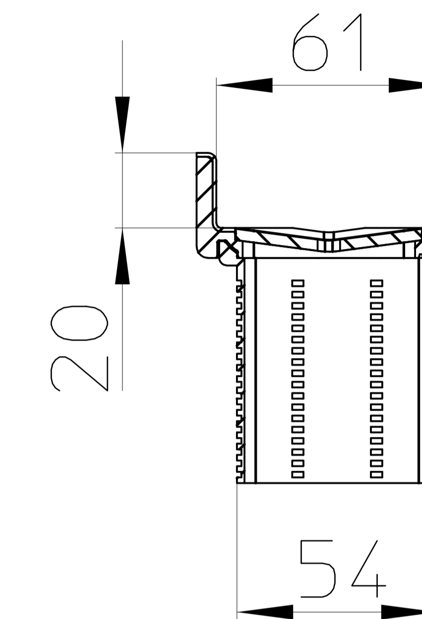
Schnitt B-B
