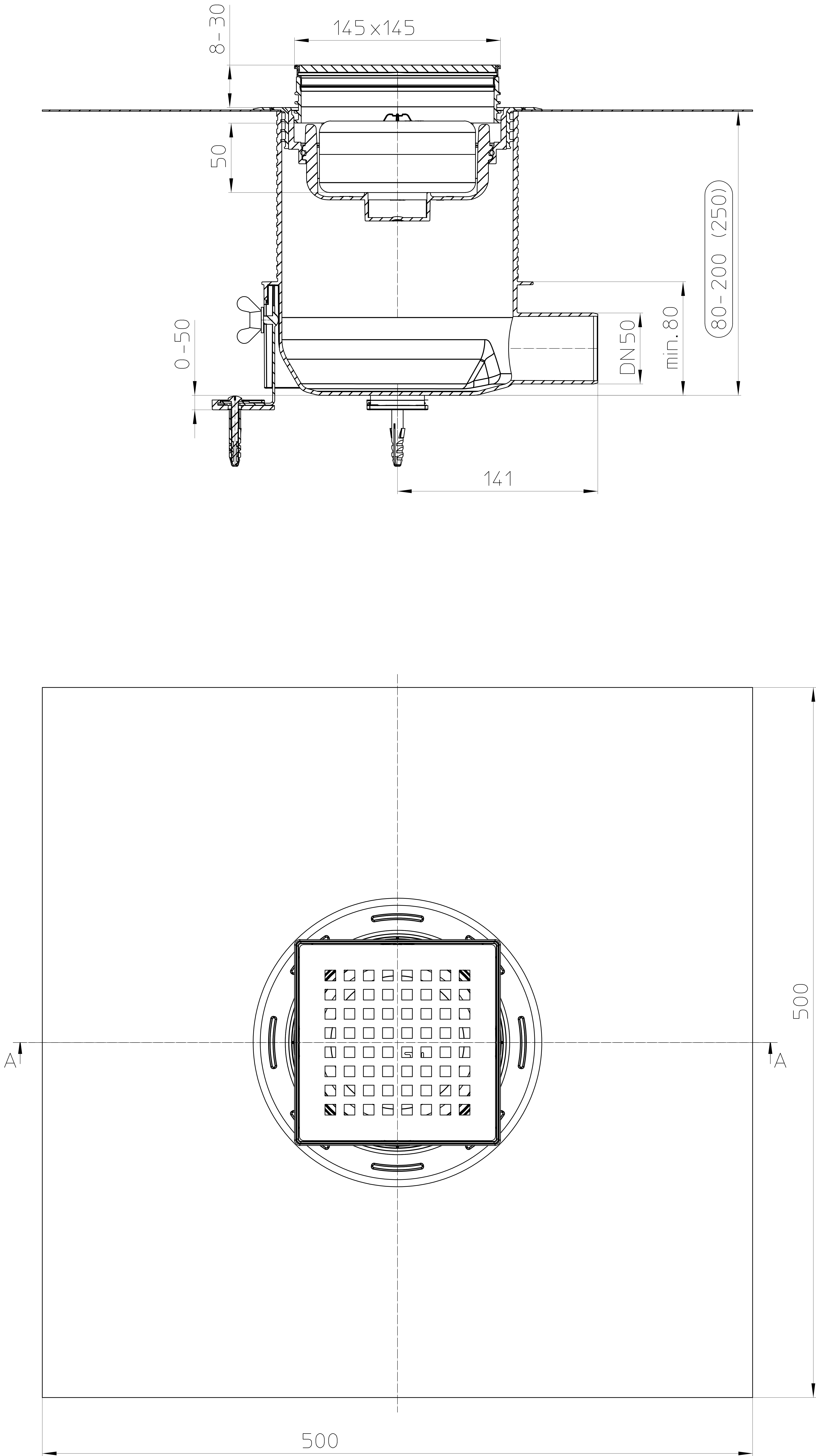
Schnitt A-A
