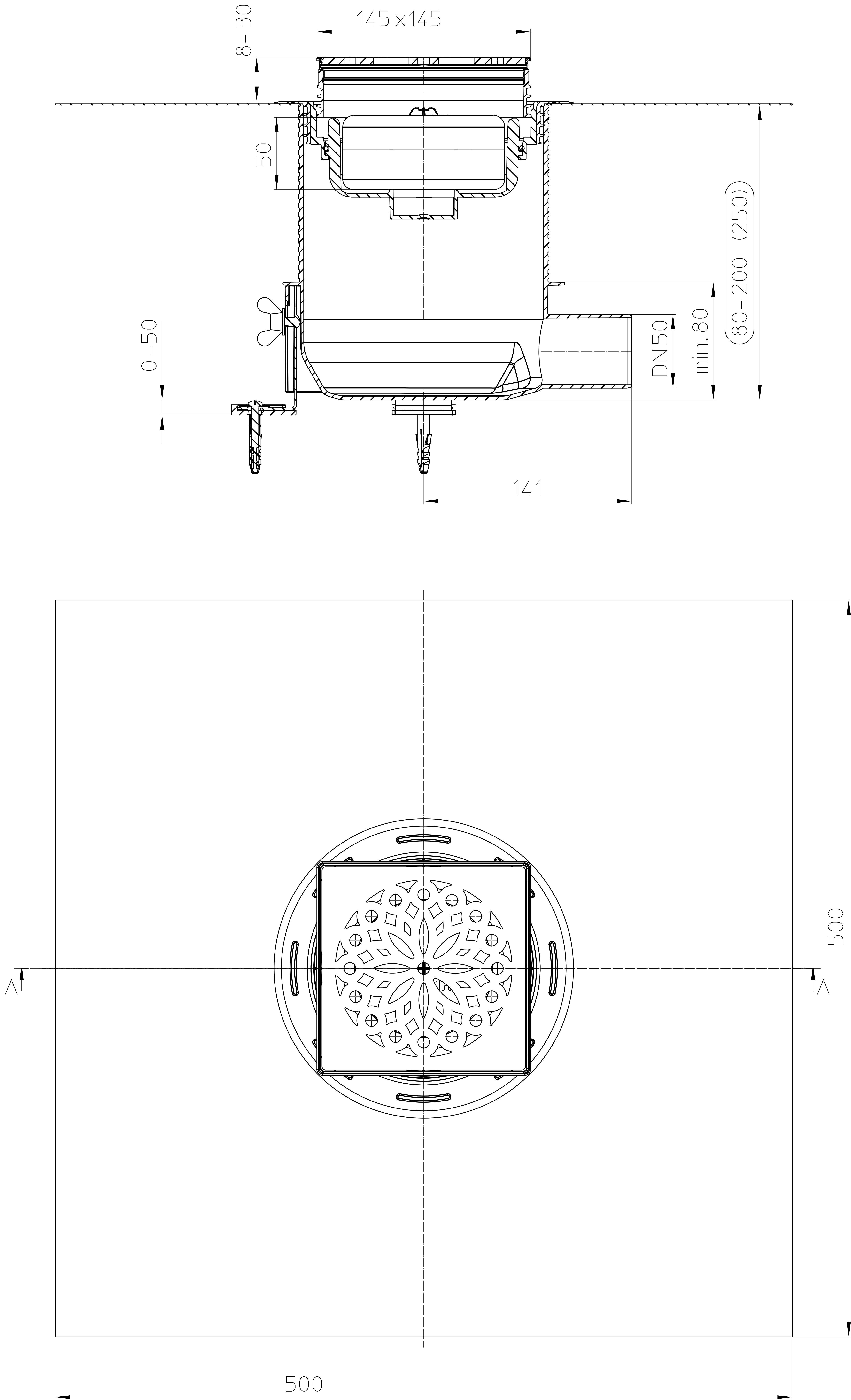
Schnitt A-A
