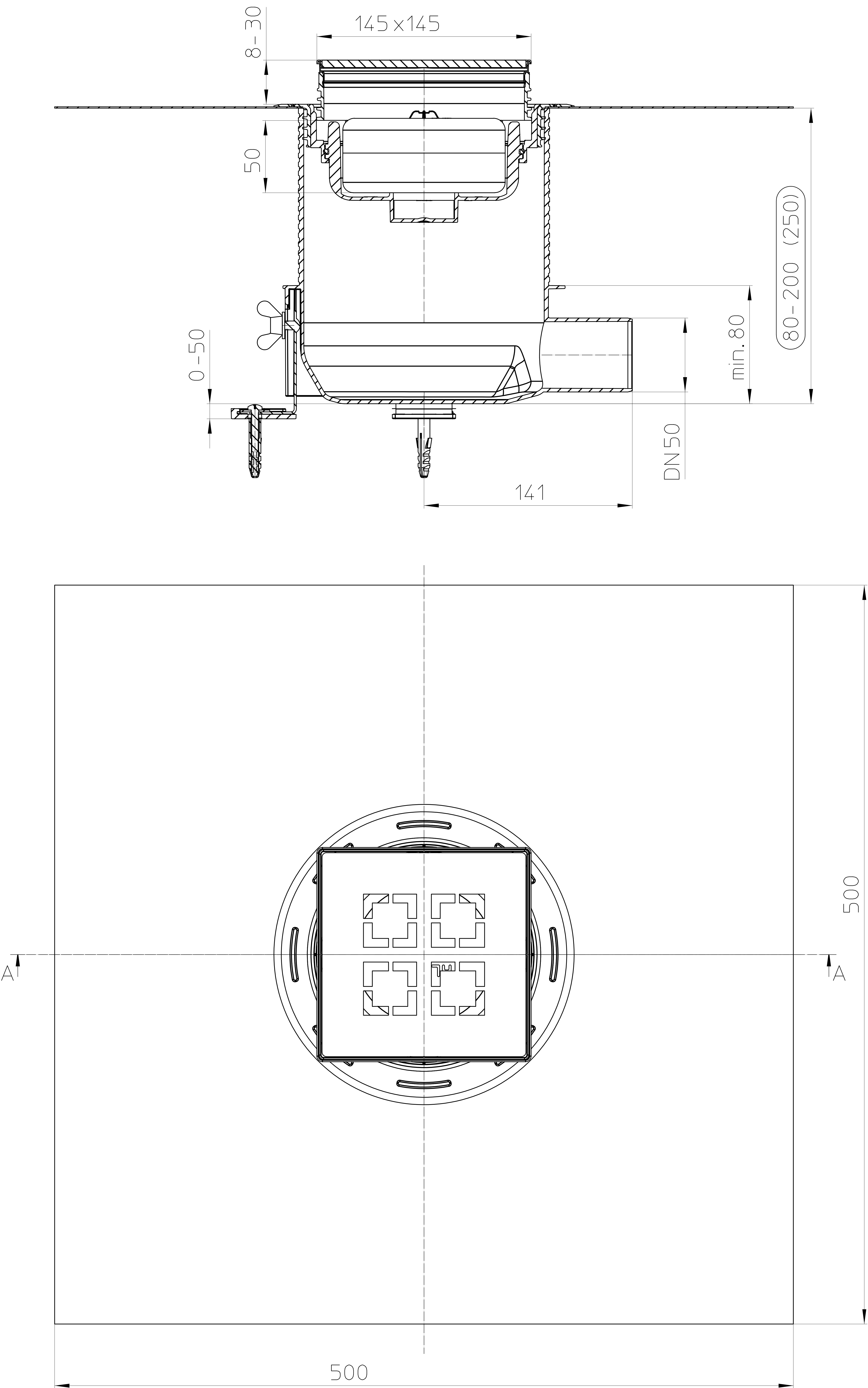
Schnitt A-A
