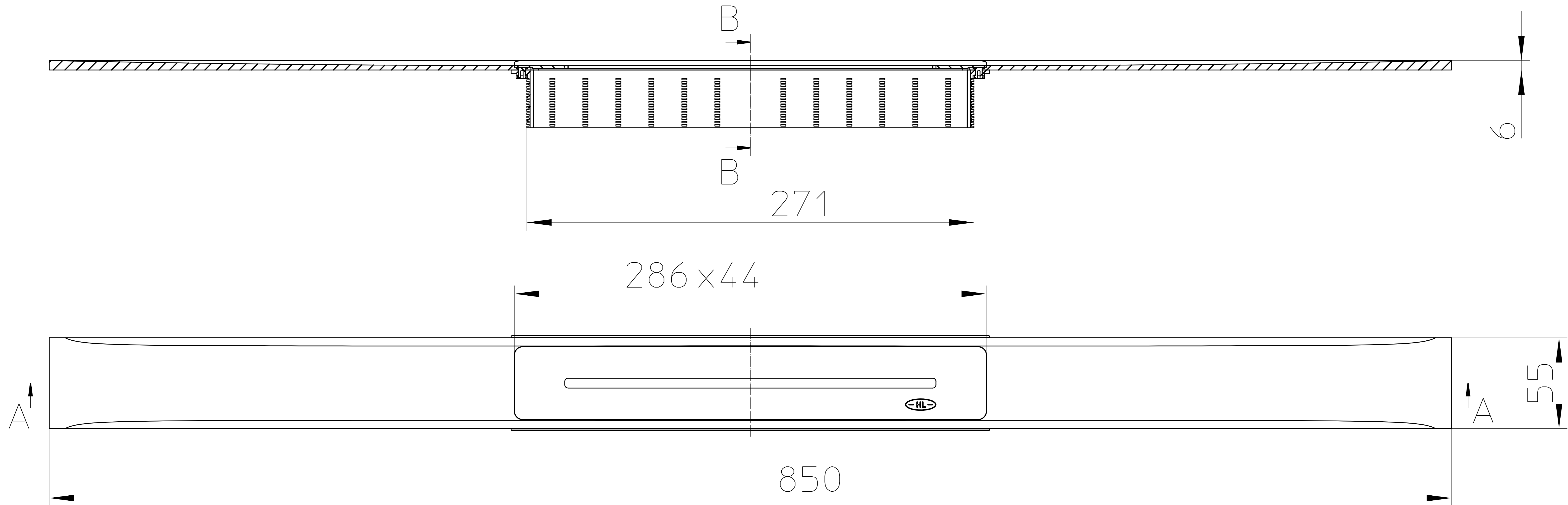
Schnitt A-A
