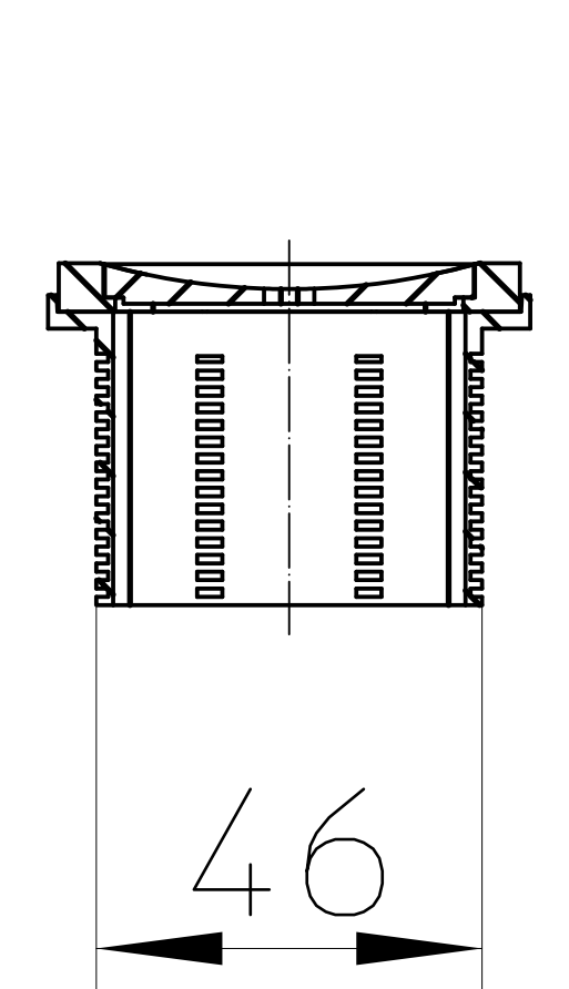
Schnitt B-B
