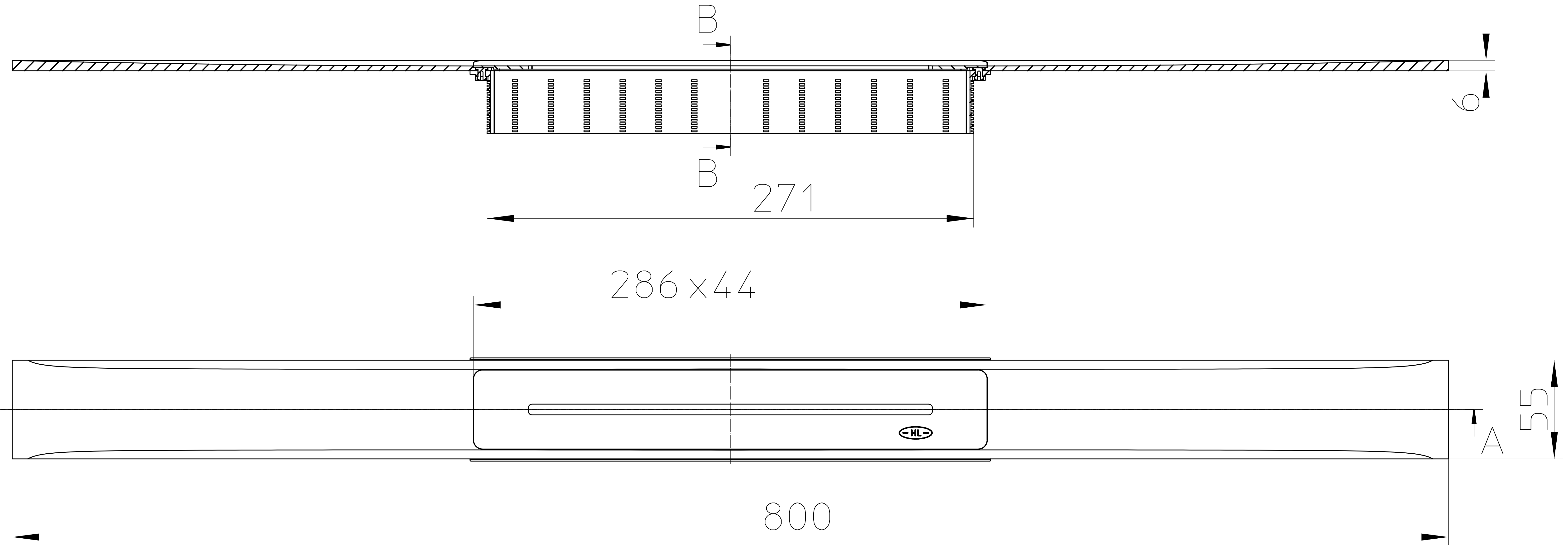
Schnitt A-A
