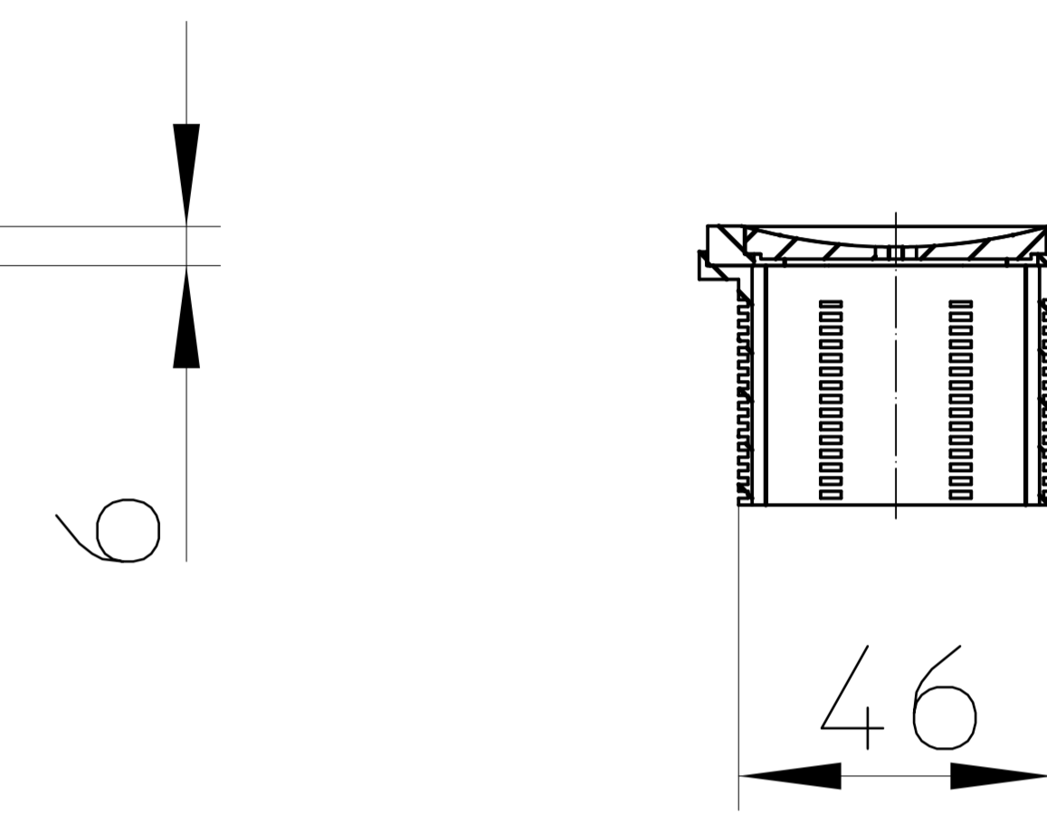
Schnitt B-B
