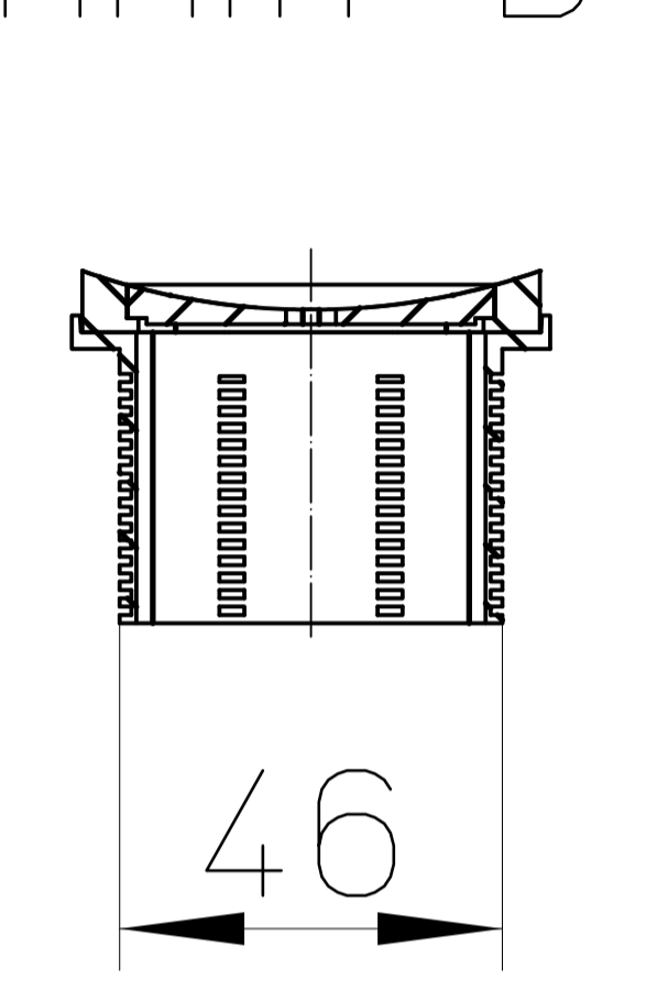
Schnitt B-B
